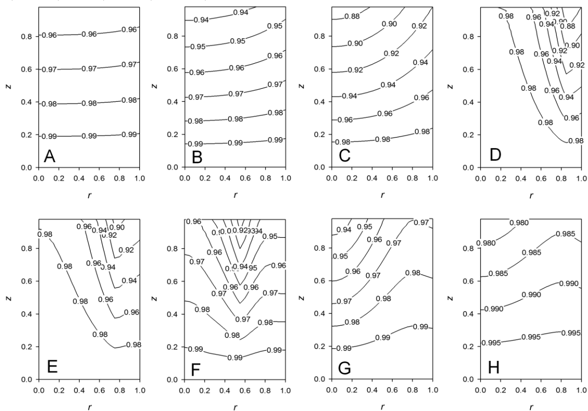
Fig. 4 Gas phase dimensionless oxygen concentration profiles for different periods. A) 2.5 h, B) 5 h, C) 10 h, D) 20 h, E) 40 h, F) 80 h, G) 140 h, H) 250 h
