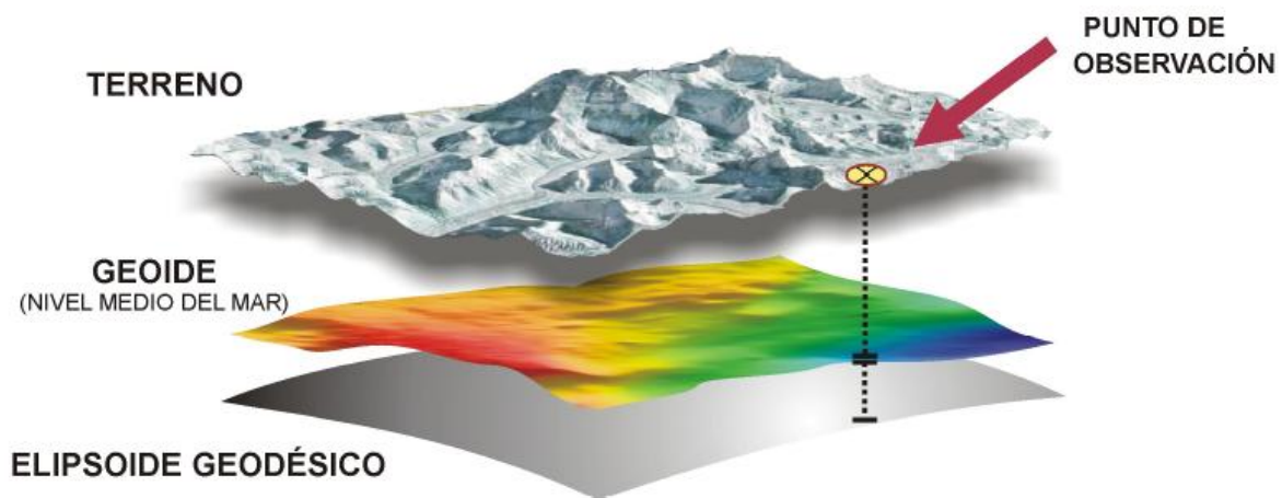
Figura 3.2: Geoide y elipsoide. INEGI (2006). MODELO GEOIDAL EN MÉXICO Y SUS APLICACIONES . [ONLINE] Available at: http://mapserver.inegi.gob.mx/geografia/espanol/normatividad/infgeodesia/ggm04/GeoideAp2006.pdf?c=713 . [Last Accessed 30 September 12].
