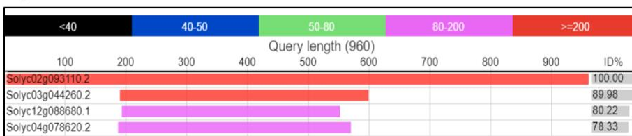
Figura 8. Alineamiento de secuencias de cDNA de SCEI y sus parálogos
