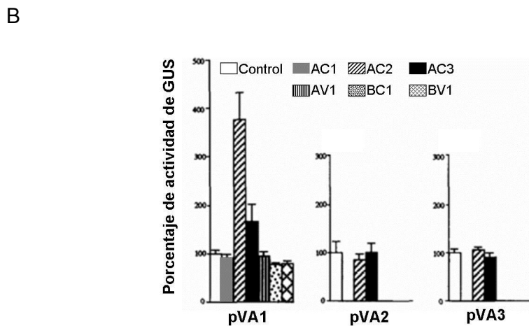
Figura 12. Ensayos de expresión transitoria utilizando diferentes versiones del promotor CP . A) Esquema de las construcciones utilizadas en el estudio B) Porcentajes de actividad del gen reportero en los ensayos de expresión transitoria en las diferentes construcciones del promotor de CP con cada una de las proteínas virales (reproducido de Haley et al., 1992)
