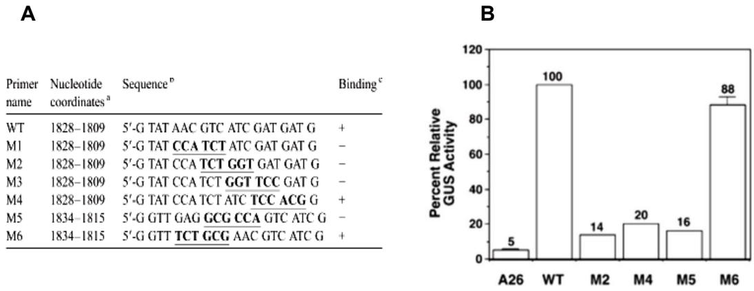
Figura 11. Mutaciones en una secuencia importante para la expresión de AC2. A) Tabla que muestra las mutaciones introducidas y su influencia en la unión específica a proteínas del hospedero B) Actividad del promotor AC2 de las construcciones con las mutaciones en la secuencia fusionada al gen reportero GUS.
