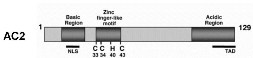
Figura 15. Diagrama de la proteína AC2. La señal de localización nuclear se encuentra localizada en el amino terminal, un motivo dedo de zinc no clásico y un dominio de activación en el carboxilo terminal. (Reproducido de Yang, 2007)
