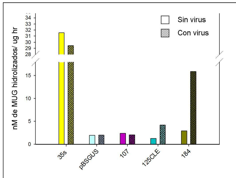
Figura 39. Resultados de la cuantificación de la actividad del GUS de diversas versiones truncadas del promotor CP de TGMV. Las barras amarillas representan los resultados del control positivo (35S-GUS), y las barras azul claro para el control negativo; en barras moradas, azul fuerte y verde se representan los resultados de las construcciones 107, 125CLE, y 184 respectivamente. Las barras vacías indican la ausencia del componente A del virus EuMV, y las barras rayadas indican su presencia.
