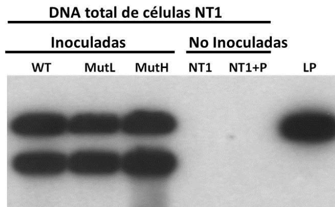
Figura 27. Análisis de la replicación viral mediante Southern blot. WT= representa al DNA obtenido de los protoplastos inoculados con el virus silvestre (PepGMV hemidimérico), MutL= Virus mutante monomérico previamente linearizado, MutH= virus mutante en forma de hemidimero. NT1= DNA de protoplastos control, NT1 + P= DNA de protoplastos con DNA viral plasmídico, LP= control positivo DNA-A linearizado.
