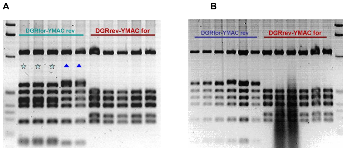
Figura 41. Patrones de restricción del componente A utilizando las enzimas EcoRI y Hinfl . A) Clonas obtenidas a partir del PCR del extracto de la planta de Sida rhombifolia , con estrellas y triángulos están señalados los dos patrones de restricción que se obtuvieron. B) Clonas obtenidas a partir del PCR del extracto de la planta de Herissantia crisper .
