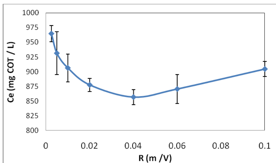
Figura 8.5 Efecto de la relación masa/volumen (m/V) en la adsorción de LS. Ce: concentración en el equilibrio.
