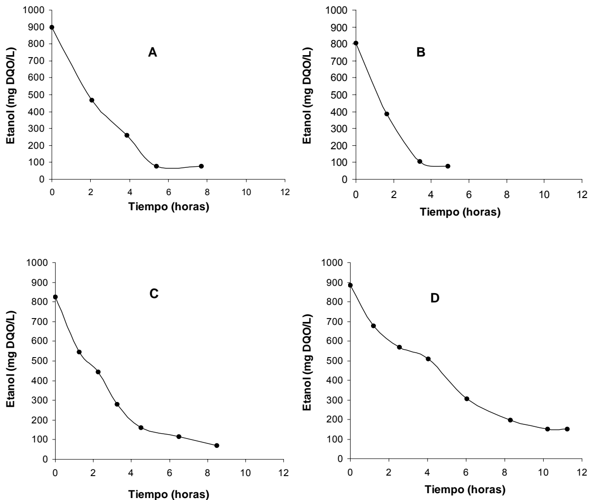
Figura 3.7 Perfiles de consumo de etanol con respecto al tiempo con sulfuro como inhibidor, para 152 mg S 2- /L (A), 255 mg S 2- /L (B), 384 mg S 2- /L (C) y 424 mg S 2- /L (D).
