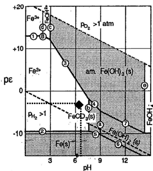
Figura 2.3 Diagrama de pE contra pH para un sistema Fe-CO 2 -H 2 O. Las fases sólidas son Fe(OH) 3 (amorfo), FeCO 3 (siderita), Fe(OH) 2 (S), y Fe(S); CT = 10 -3 M. Las líneas son calculadas para Fe(II) y Fe(III) = 10 -5 M (25°C) (Stumm y Morgan, 1996).
