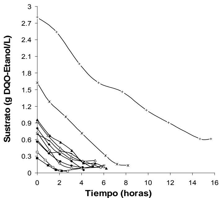
Figura 3.4 Cinéticas del consumo de DQO con respecto al tiempo con etanol como sustrato (g DQO-etanol/L): 0.26 (■), 0.37 (□), 0.55 (●), 0.59 (○), 0.69 (-), 0.72 (◇), 0.80 (◆), 0.92 (△), 0.96 (▲), 1.62 (*) y 2.8 (+).
