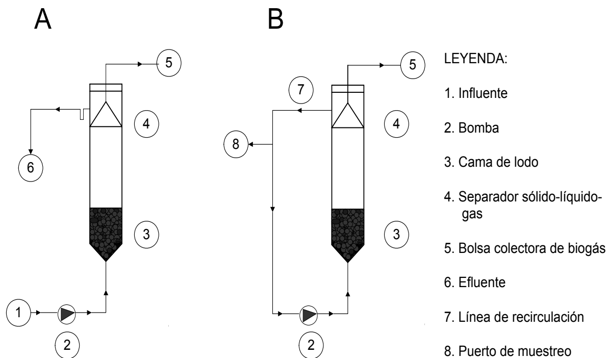
Figura 2.1 Representación esquemática del reactor UASB operado en flujo continuo (A) y operado en lote (B).
