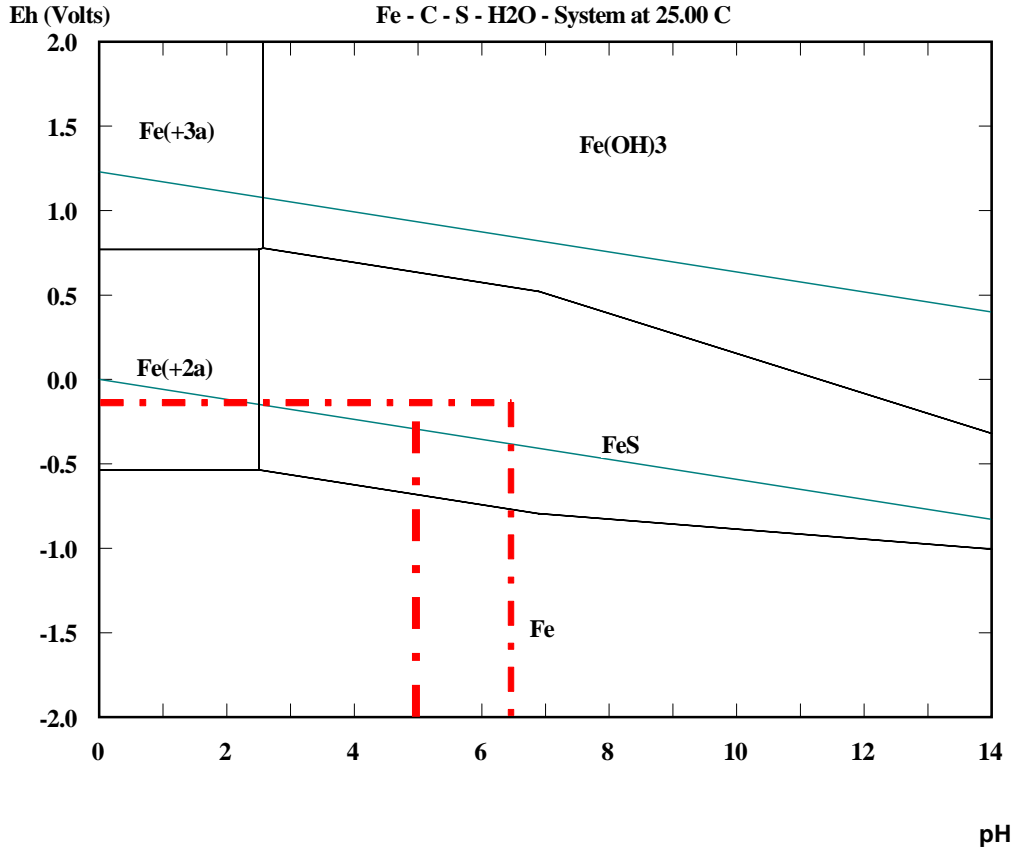
Figura 3.11 Diagrama de potencial redox (Eh) contra pH para un sistema Fe C-S-H 2 O. Las fases sólidas son Fe(OH) 3 , y Fe(S). La fase sólida de FeCO 3 no fue significativa.
